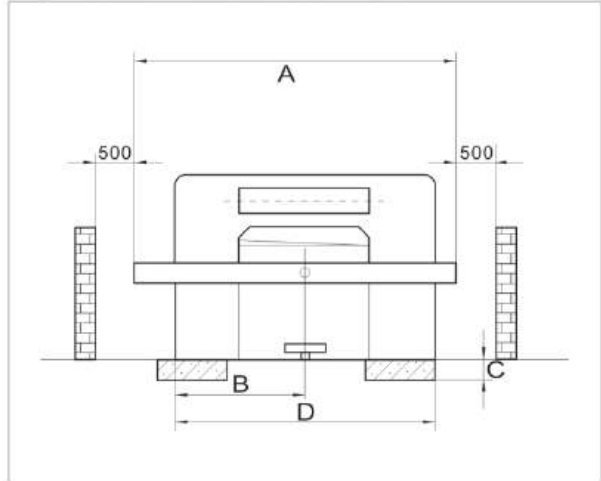
安装尺寸 Installation dimension
